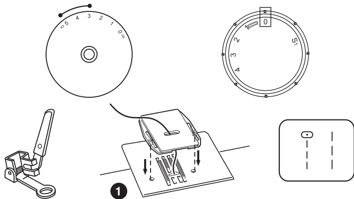
Ручка выбора ширины строчки
